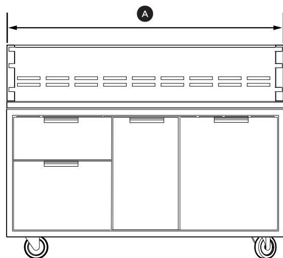
CAD1-48/48E Vue de face
