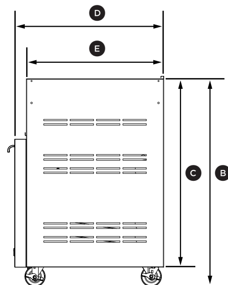
CAD1-30, CCAD1-36/36E and CAD1-48/48E Vue de côté
